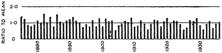
टेन, चट्टानगा पर टेनेसी नदी (औसत, २४.३४ इंच। समय १८७५-१९३६)
